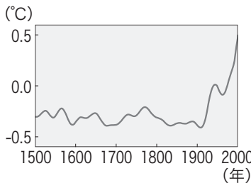
過去500年間の気温の変化
