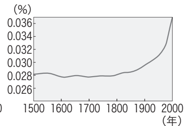
過去500年間の空気中にふくまれる二酸化炭素の体積の割合の変化
